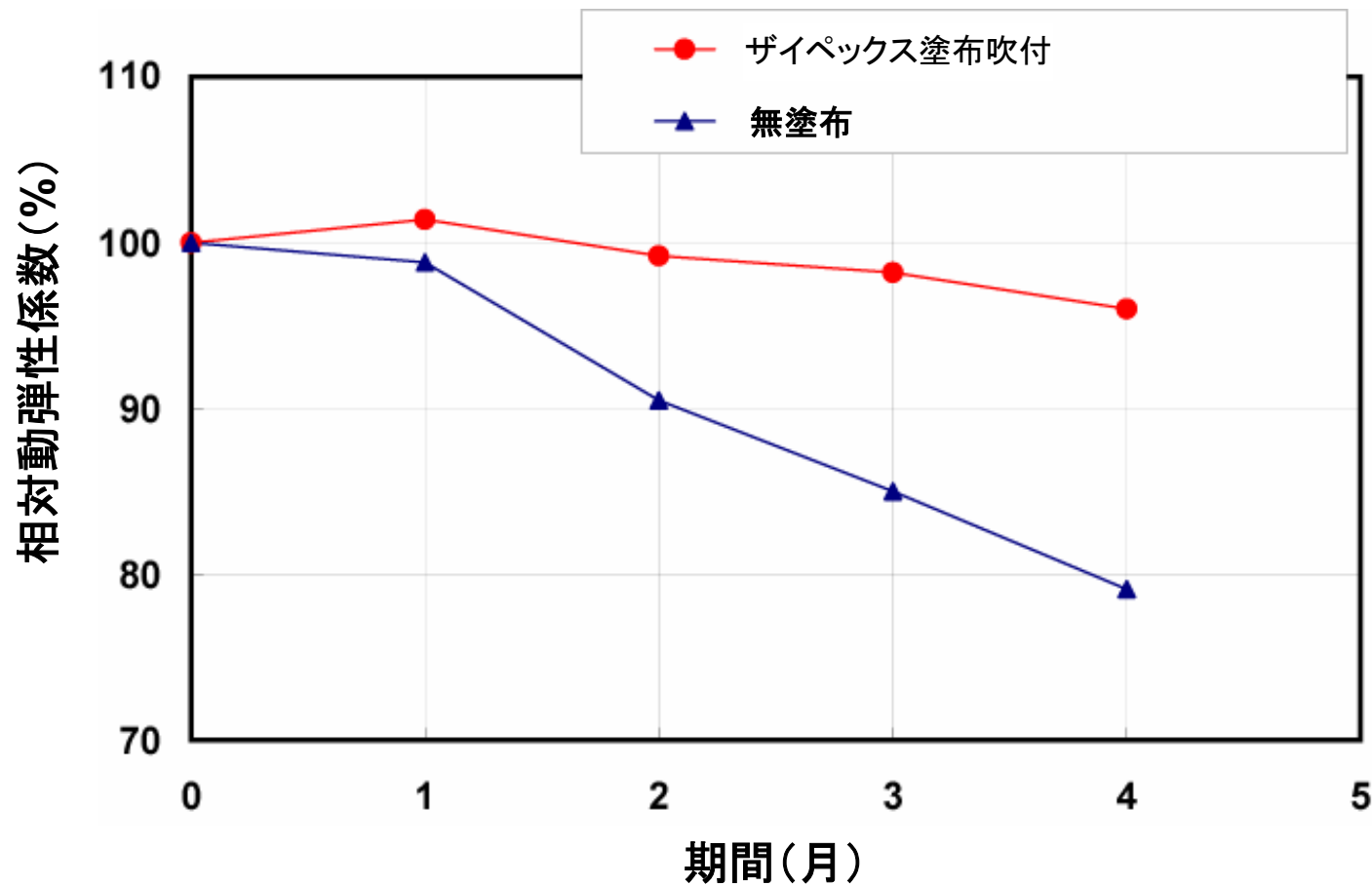
耐酸性コンクリートの性能試験
